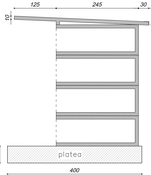
COPERTURA B
