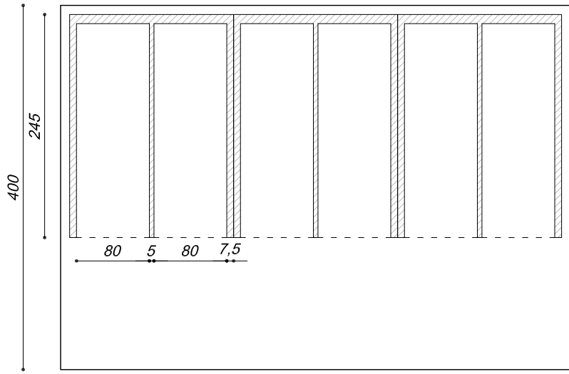
PIANTA/PLATEA
