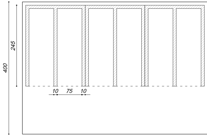
VISTA FRONTALE
