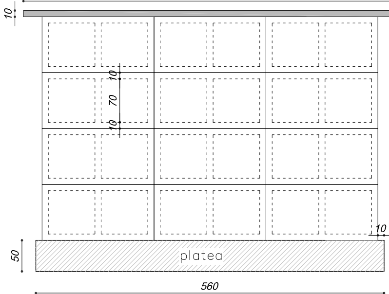
VISTA FRONTALE
