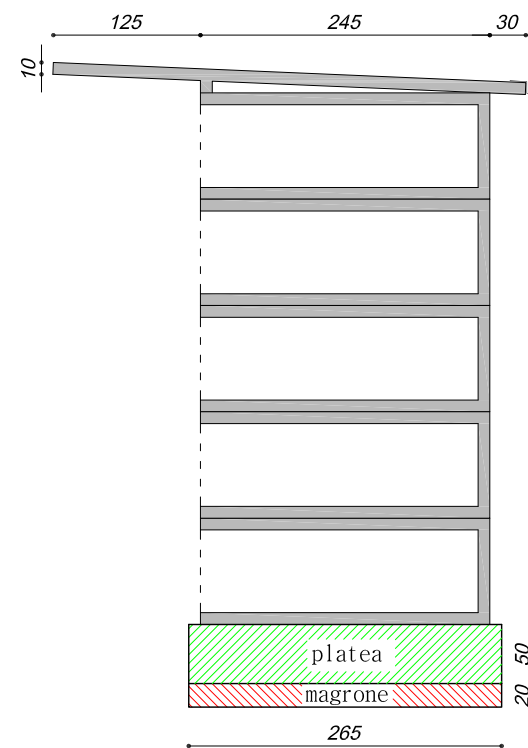
VISTA SEZIONE
