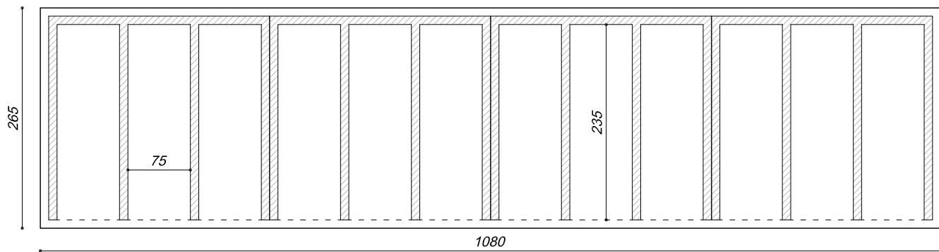
PIANTA/PLATEA
