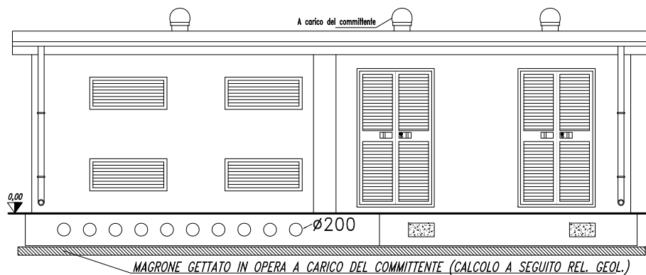
PROSPETTO A
