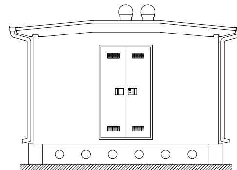
PROSPETTO D
